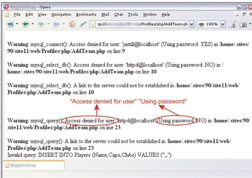
Figura 8. Error de la base MySQL
