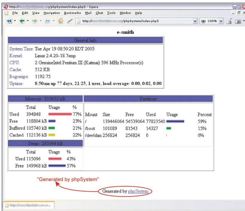
Figura 5. Estadísticas de phpSystem
