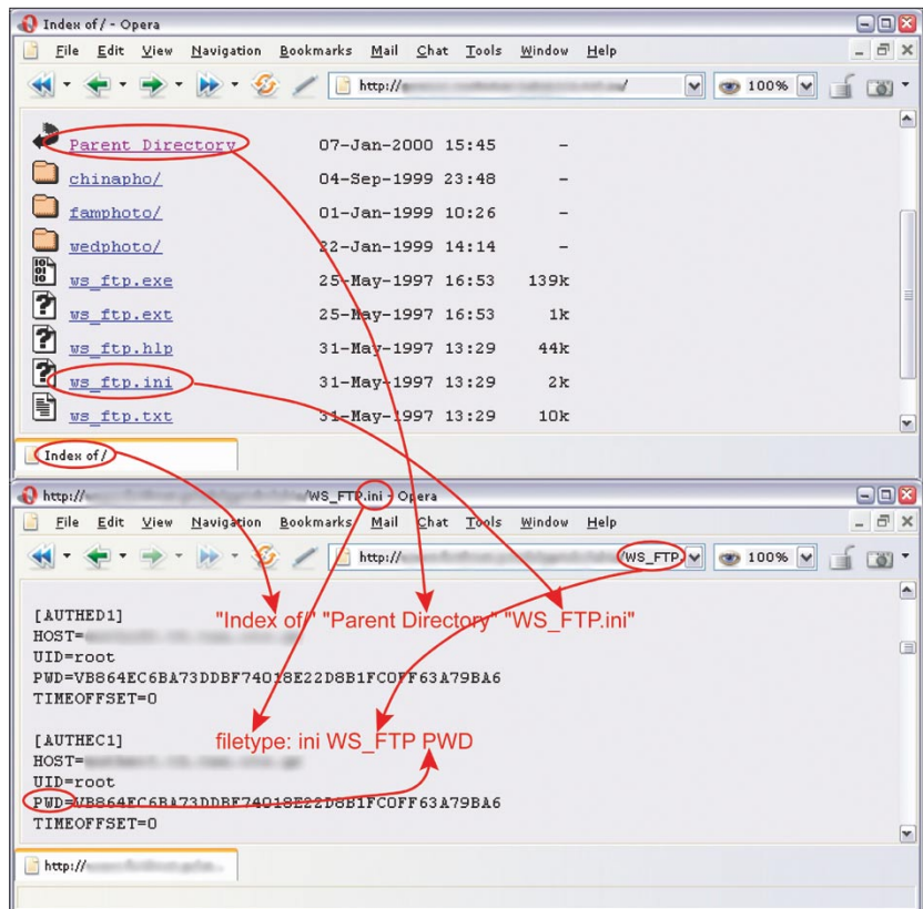
Figura 9. Fichero de configuración del programa WS_FTP
