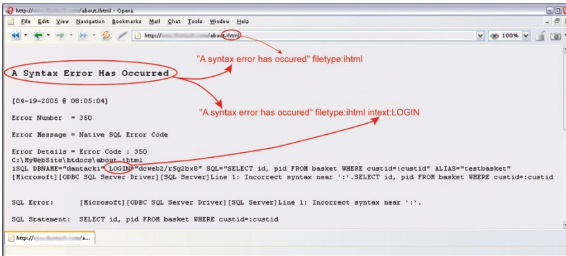
Figura 7. Modos de aprovecharse de errores en la base de datos Informix
