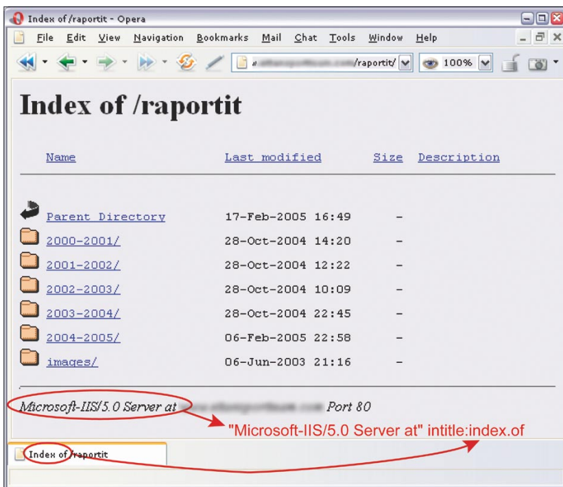
Figura 2. La detección del servidor IIS 5.0 con el uso del operador intitle
