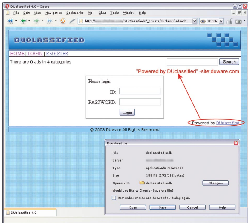
Figura 10. Programa DUclassified , configurado de modo estándar
